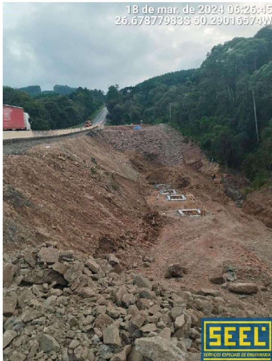
8.3.9 – Aterro da drenagem profunda.
