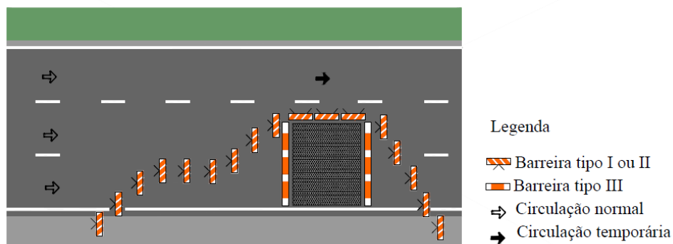
Figura 7.: Esquema de utilização de barreiras Tipo I, II e III
