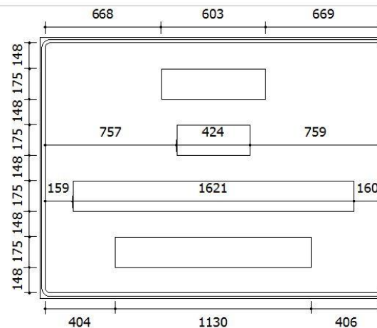
Figura 131.: Pista sem acostamento a 200 m
