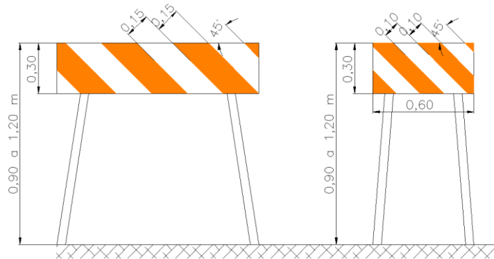
Figura 10.: Barreiras Tipo I (horizontal)
