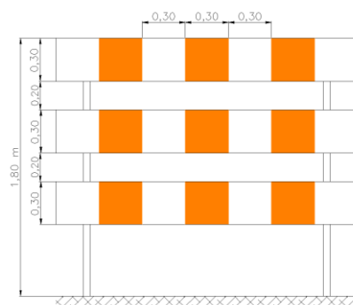
Figura 13.: Barreira Tipo III
