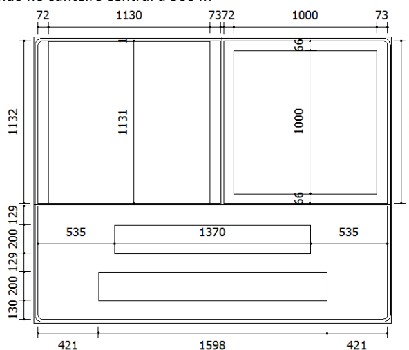
Figura 164.: Placa composta A-24 + R-7 + "Reduza a Velocidade"
