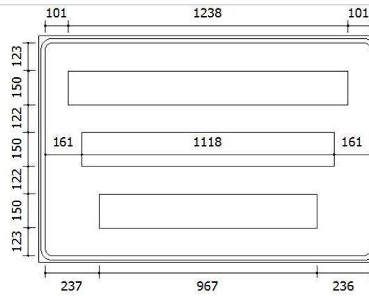
Figura 129.: Tráfego em meia pista a 500 m
