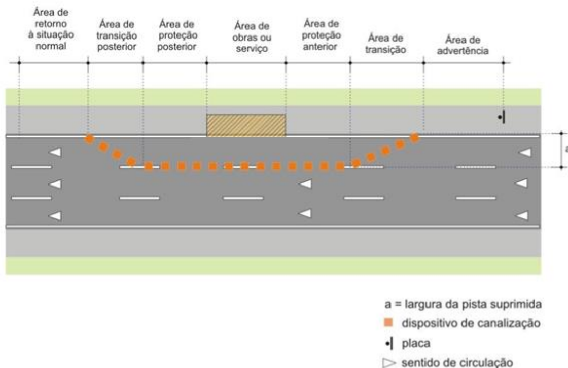
Figura 3.: Zona de Controle de Tráfego
