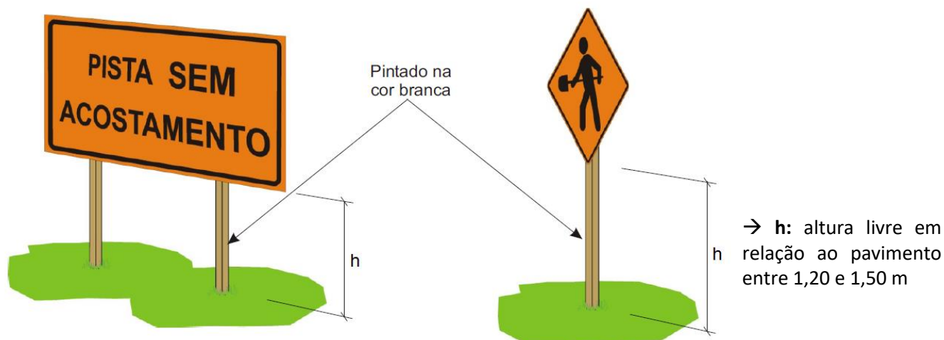
Figura 17.: Placas em pontalete de madeira
