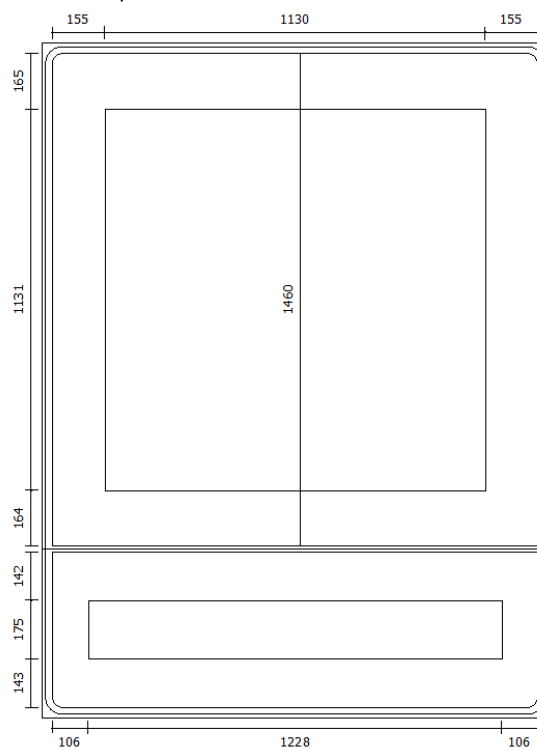
Figura 137.: Estreitamento de Pista à Esquerda a 500 m
