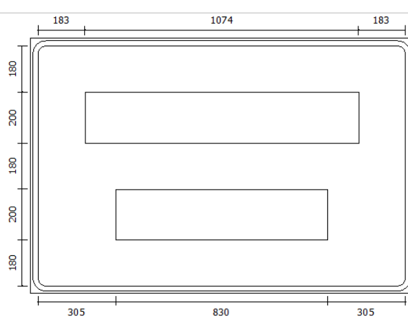
Figura 132.: Fim das Obras
