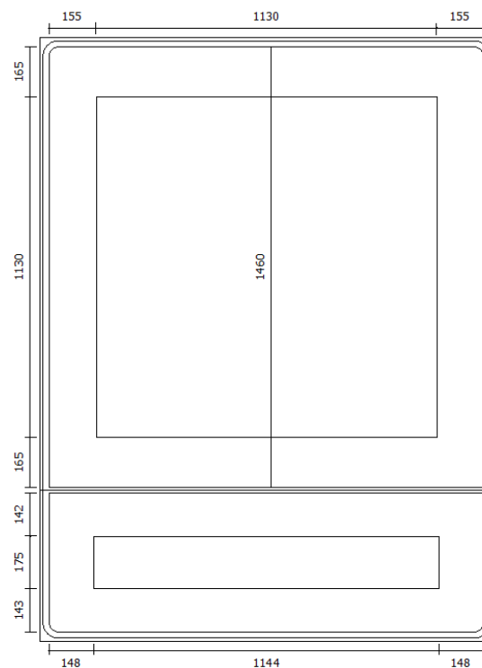
Figura 145.: Pista Dividida a 100 m
