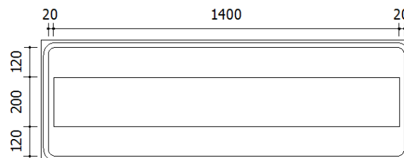
Figura 168.: Placa complementar "A 200 m"
