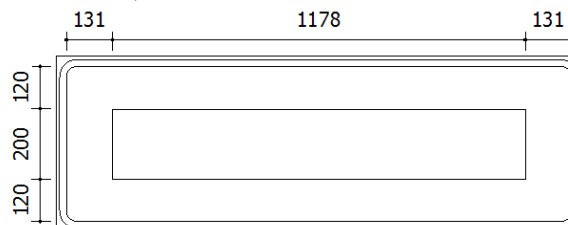
Figura 173.: Placa complementar "A 1,5 km"
