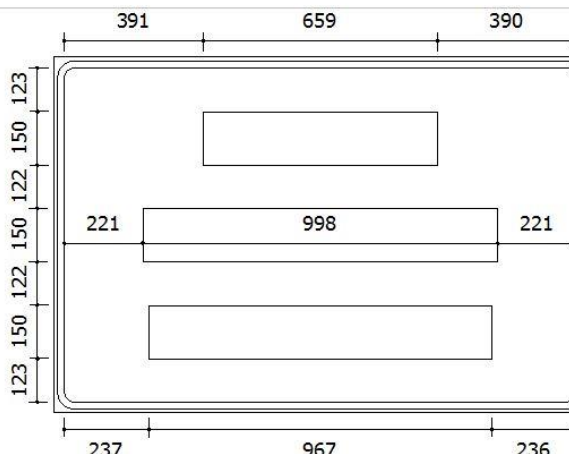
Figura 112.: Desvio à direita a 200 m
