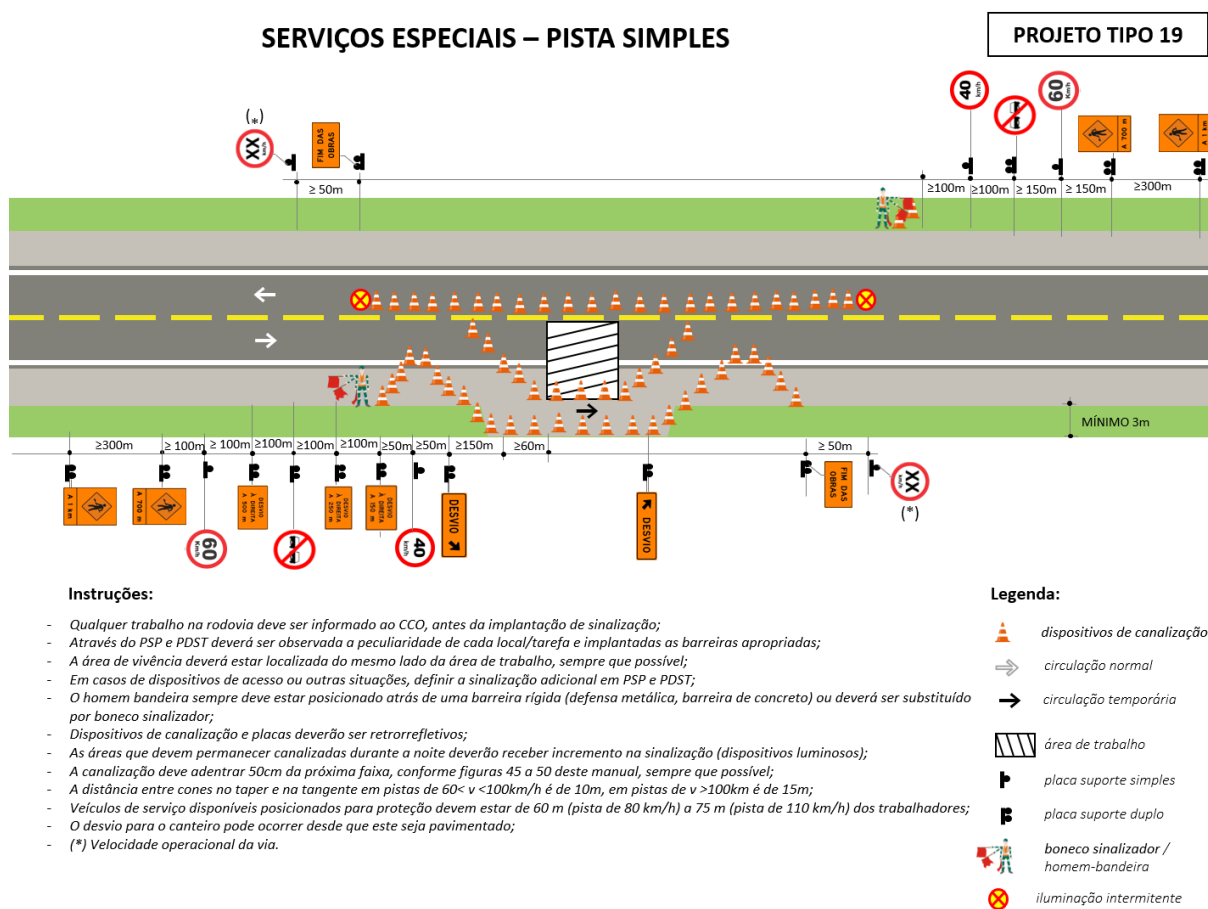
Figura 77.: Serviços especiais– pista simples
