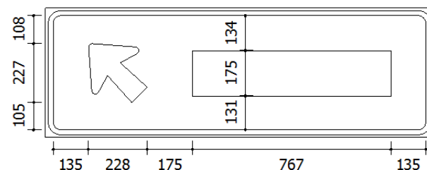
Figura 109.: Desvio à esquerda
