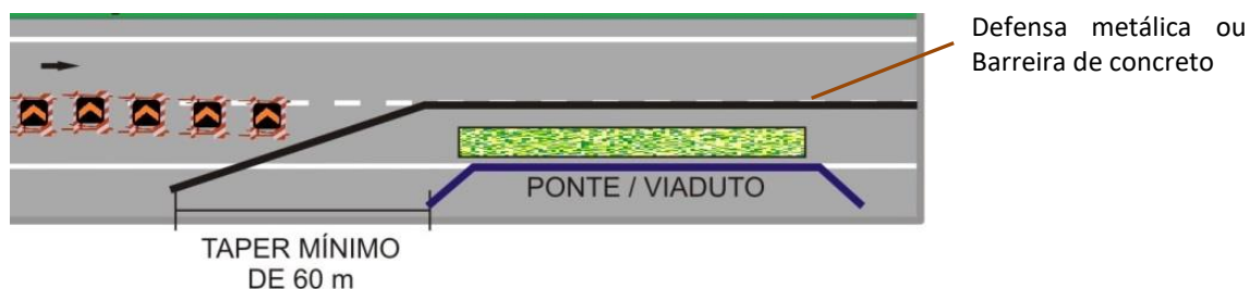
Figura 34.: Exemplo de Uso de Barreira Provisória em Obra de Recuperação/alargamento de pontes e/ou viaduto
