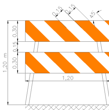
Figura 12.: Barreira Tipo II
