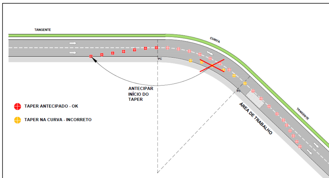
Figura 1.: Antecipação da sinalização em curvas horizontais
