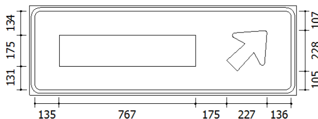
Figura 108.: Desvio à direita
