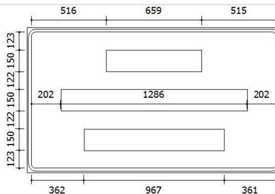
Figura 121.: Desvio à esquerda a 300 m
