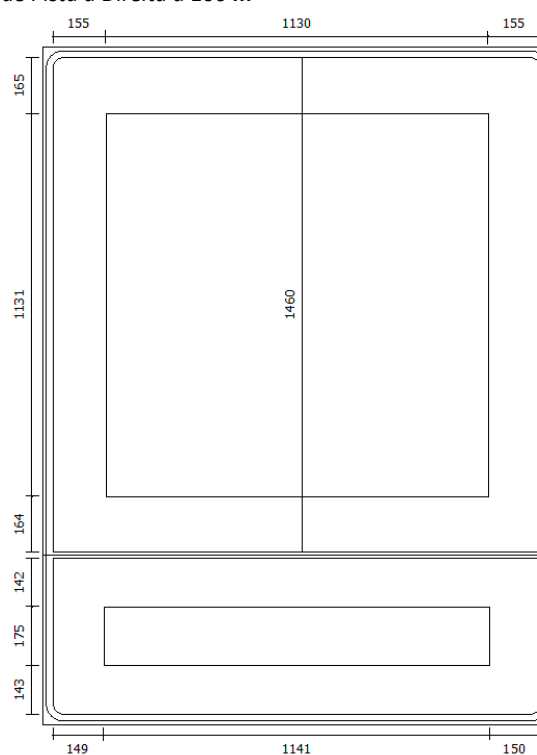
Figura 139.: Estreitamento de Pista à Direita a 150 m
