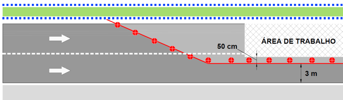
Figura 46.: Posicionamento de dispositivos de canalização – Pista com 2 Faixas (caso 2)
