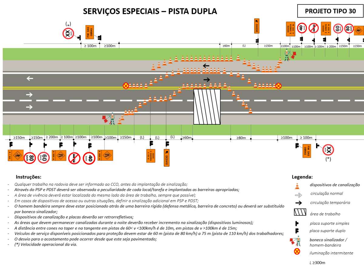
Figura 88.: Serviços especiais– pista dupla
