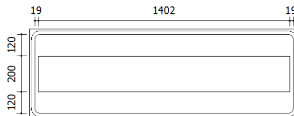
Figura 167.: Placa complementar "A 150 m"
