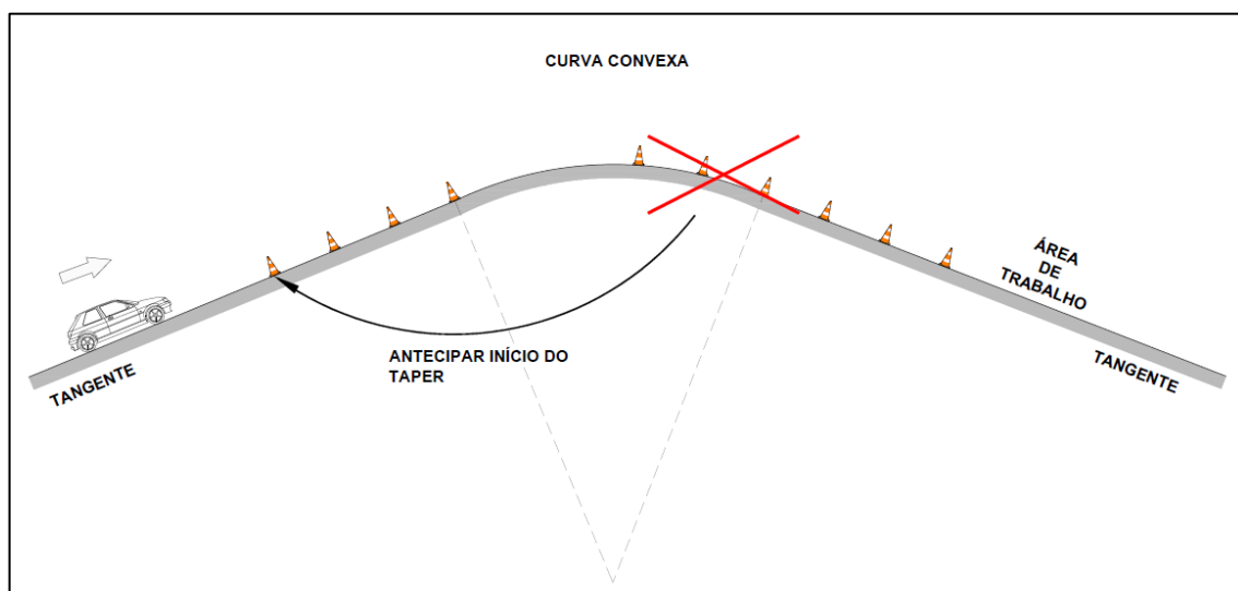
Figura 2.: Antecipação de sinalização em curvas verticais convexas
