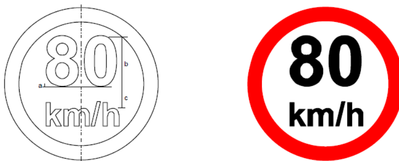
Figura 95.: Placa R-19 (Velocidade Máxima Permitida)
