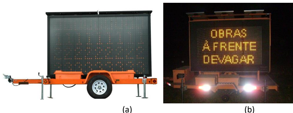
Figura 25.: Painel de mensagem variável móvel: (a) ilustração, (b) painel em utilização
