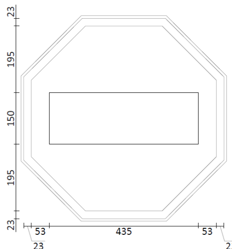
Figura 101.: Placa SIGA para procedimento "PARE e SIGA"
