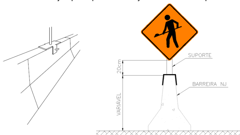
Figura 15.: Suporte tipo jacaré
