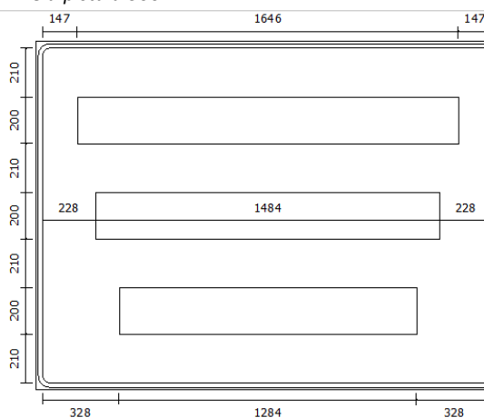
Figura 130.: Tráfego em meia pista a 700 m
