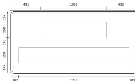
Figura 104.: Obras a 1000 m
