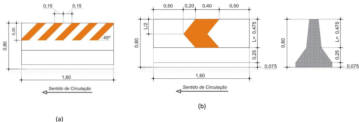
Figura 35.: Elementos/pintura para sinalização das barreiras provisórias
