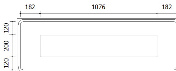
Figura 171.: Placa complementar "A 700 m"
