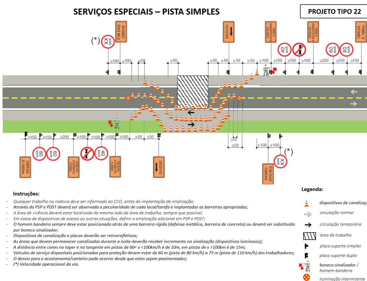
Figura 80.: Serviços especiais– pista simples
