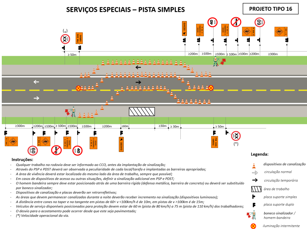
Figura 74.: Serviços especiais– pista simples
