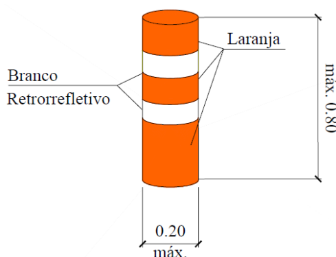
Figura 29.: Cilindro delimitador
