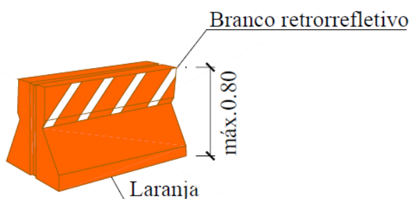
Figura 28.: Barreira plástica
