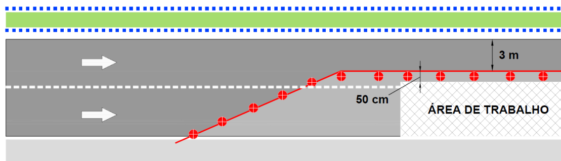
Figura 45.: Posicionamento de dispositivos de canalização – Pista com 2 Faixas (caso 1)
