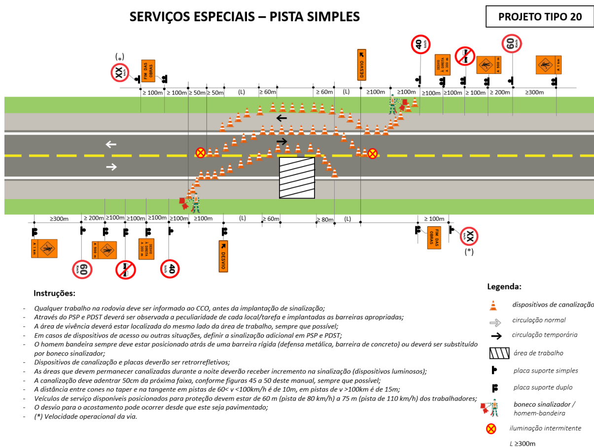
Figura 78.: Serviços especiais– pista simples
