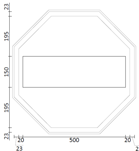
Figura 100.: Placa PARE para procedimento "PARE e SIGA"
