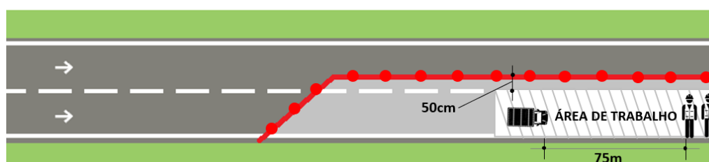
Figura 31.: Posicionamento de veículos disponíveis (velocidade normal de via 110km/h)
