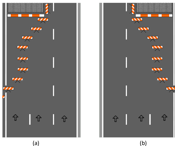
Figura 9.: Sentido das tarjas oblíquas das barreiras Tipo I, II e III para sinalização de obras do: lado esquerdo (a) e direito (b) da via
