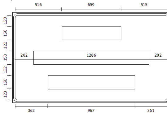
Figura 119.: Desvio à esquerda a 200 m
