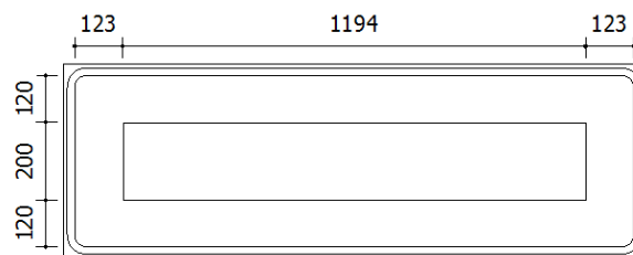
Figura 165.: Placa complementar "A 50 m"
