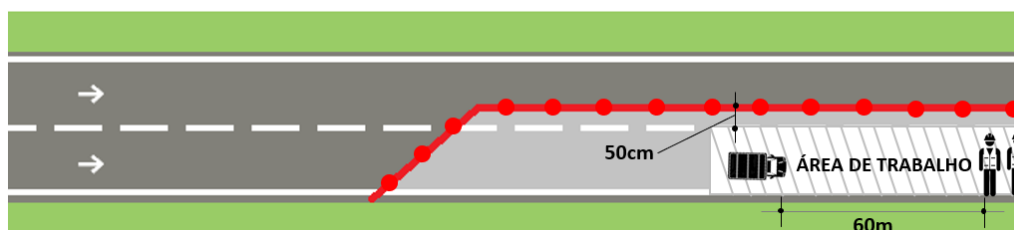
Figura 30.: Posicionamento de veículos disponíveis (velocidade normal de via 80km/h)
