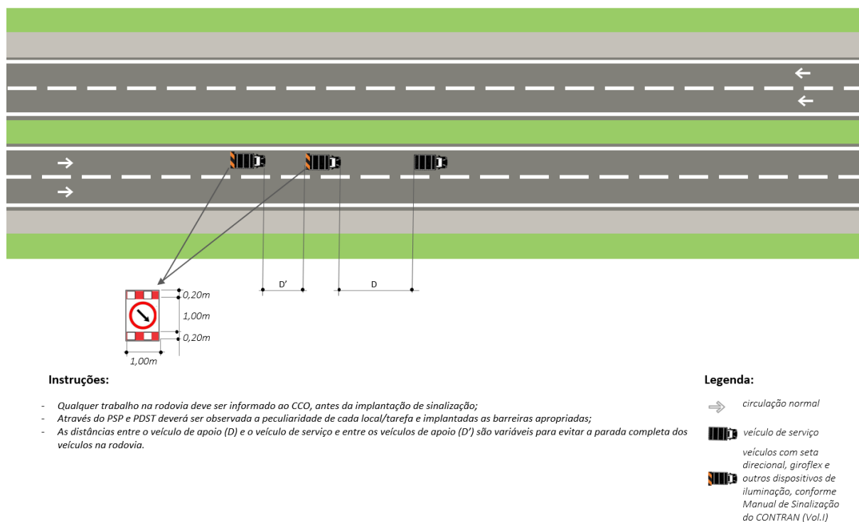
Figura 72.: Serviço na faixa 1 de rolamento – pista dupla
